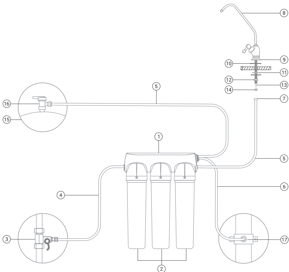
Рис. 11. Схема подключения Престиж Смарт.
