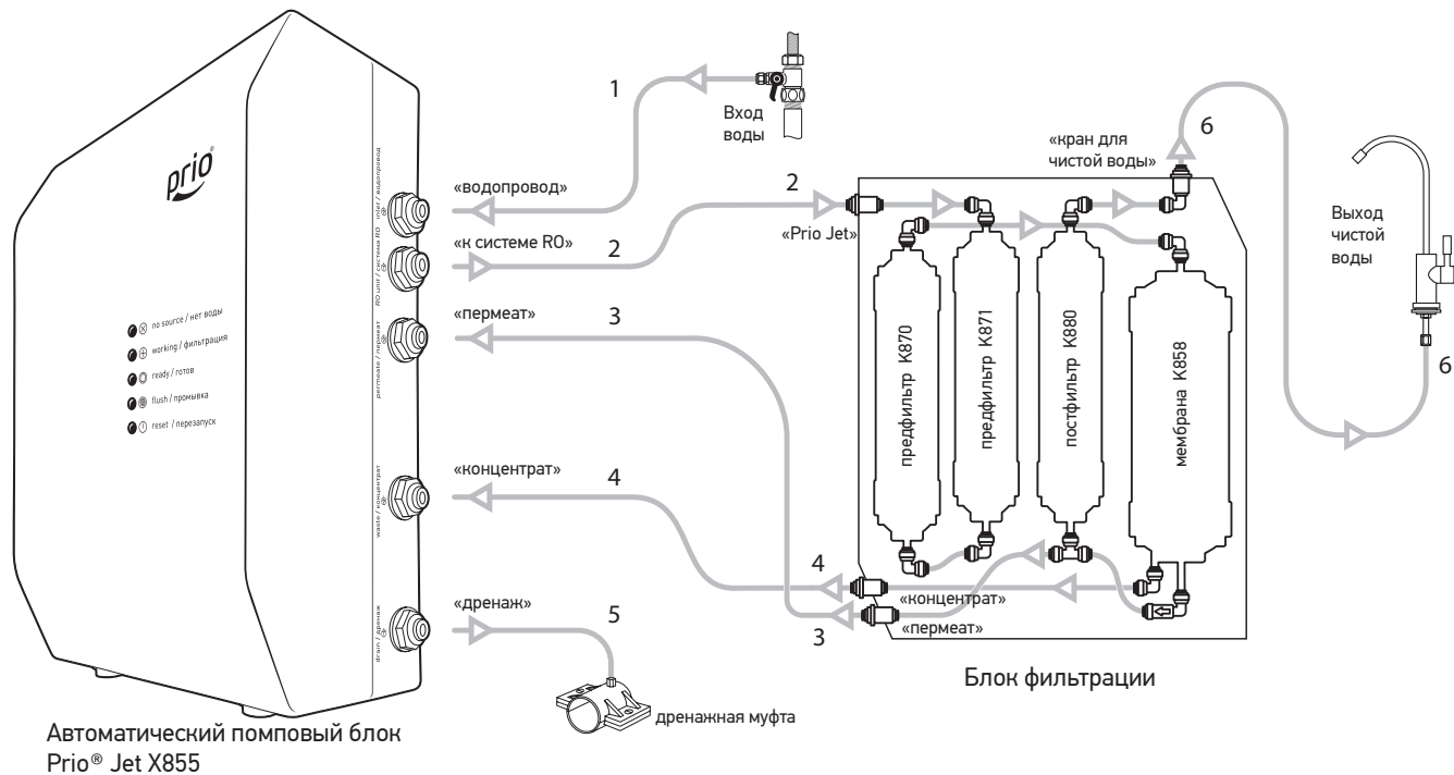
Рис.2. Принципиальная схема подключения системы Expert Osmos Stream MOD600
