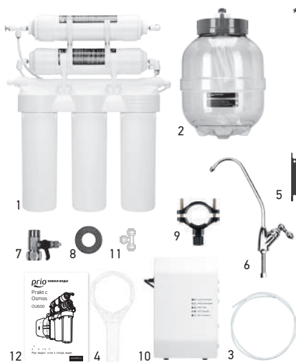
Рис.3. Комплект поставки фильтра Praktic Osmos.
